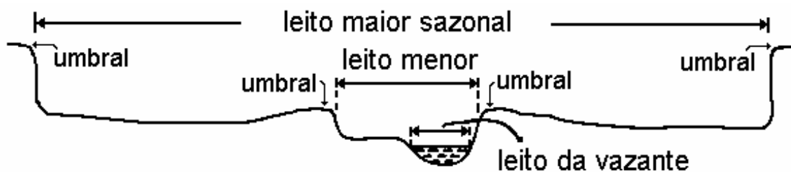
Figura 1 – Tipos de leitos fluviais em planícies de inundação
