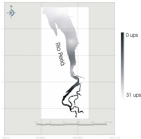
Figura 2 - Salinidade do Estuário durante a maré cheia.
