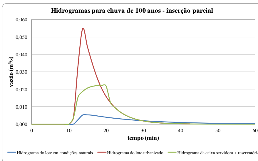
Figura 5 – Hidrograma do reservatório de detenção de 2,0 m 3 com chuva parcial
