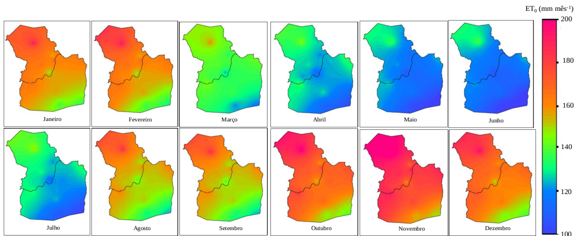
Figura 3 – Mapas dos valores médios da evapotranspiração de referência ( ET_0 ) para diferentes meses do ano nos municípios de Petrolina-PE e Juazeiro-BA.
