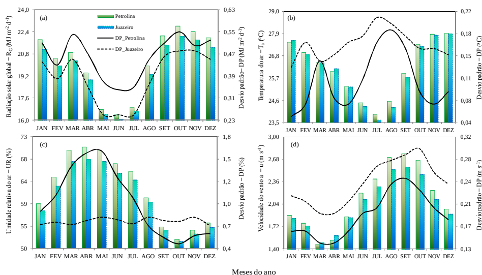
Figura 2 – Valores médios mensais e desvios padrões (DP) para as variáveis representativas da demanda atmosférica do período de 2003 a 2012 nos municípios de Petrolina-PE e Juazeiro-BA. (a) Radiação solar global – R_G ; (b) Temperatura média do ar – T_a ; (c) Umidade relativa média do ar – UR; e (d) Velocidade média do vento a 2m de altura – u .
