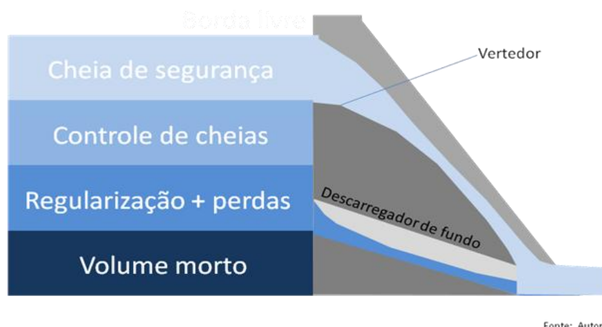
Figura 1 – Volumes de uma barragem. Fonte: Autor
