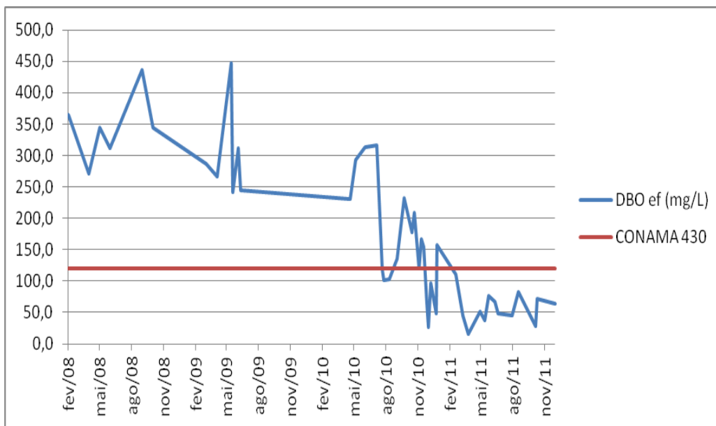
Figura 1: Gráfico do Efluente Final
