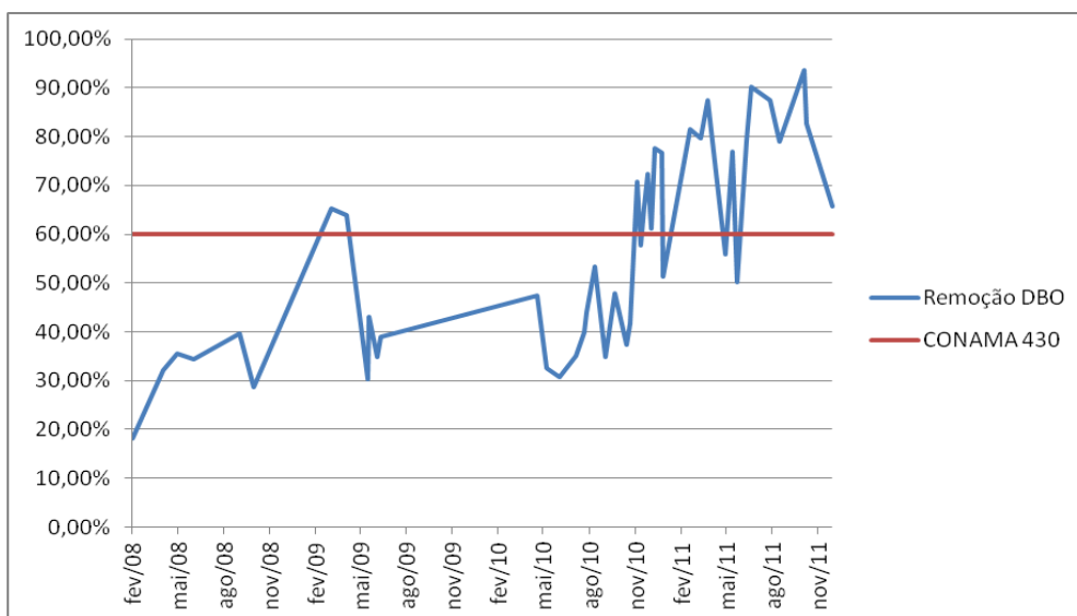
Figura 2: Gráfico de Eficiência na Remoção de DBO
