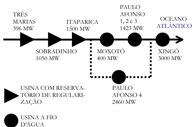
Figura 1 - Esquema Topológico do São Francisco
