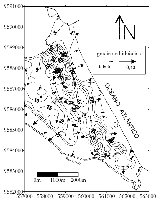
Figura 4 – Mapa de linhas isotopociais com vetores indicando direção e sentido do fluxo subterrâneo.
