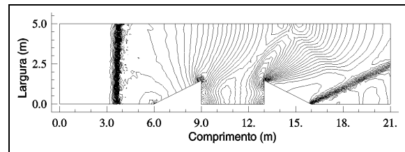
Figura 15. Isolinhas da profundidade total d'água.
