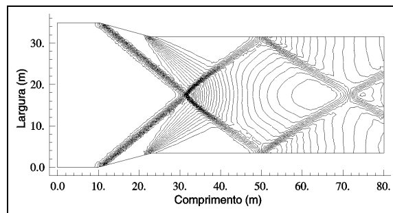
Figura 5. Isolinhas da profundidade total d'água.
