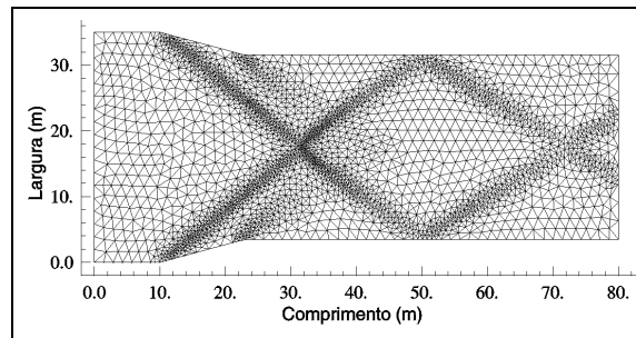
Figura 4. Malha refinada, contendo 3152 nós e 6137 elementos.
