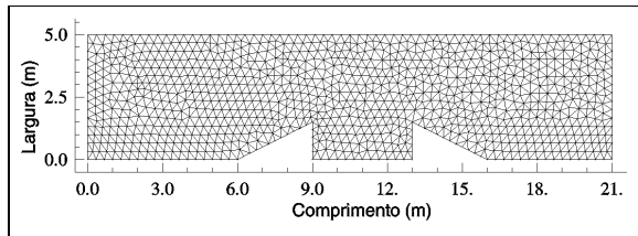
Figura 7. Domínio computacional discretizado com 1010 nós e 1849 elementos.
