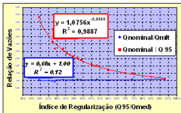
Figura 2 – Relação de vazões em função do índice de regularização.
